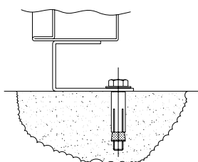
SUGESTÃO DE CHUMBADOR CHUMBADOR Ø3/8"
