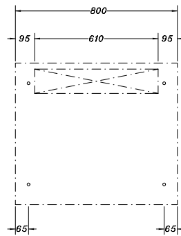
PLANTA PARA LOCALIZAÇÃO DE FIXAÇÃO, ENTRADA E SAÍDA DE CABOS, PARA COLUNAS COM COMPARTIMENTO PARA CABOS
