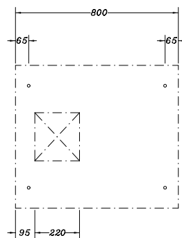
PLANTA PARA LOCALIZAÇÃO DE FIXAÇÃO, ENTRADA E SAÍDA DE CABOS, PARA COLUNAS SEM COMPARTIMENTO PARA CABOS
