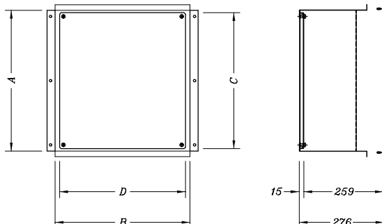
Caixa de medição para coluna de entrada
