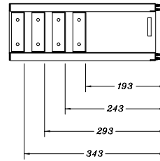
COLUNA DE DISTRIBUIÇÃO SEM COMPARTIMENTO PARA CABOS
