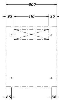
PLANTA PARA LOCALIZAÇÃO DE FIXAÇÃO, ENTRADA E SAÍDA DE CABOS, PARA COLUNAS COM COMPARTIMENTO PARA CABOS
