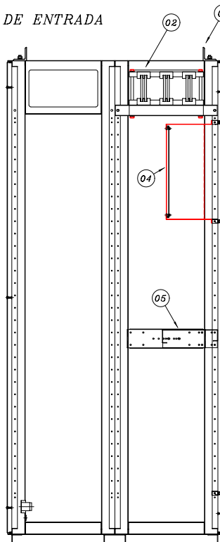
CORTE LATERAL
