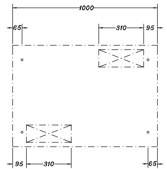
PLANTA PARA LOCALIZAÇÃO DE FIXAÇÃO, ENTRADA E SAÍDA DE CABOS, PARA COLUNAS COM COMPARTIMENTO PARA CABOS
