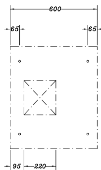
PLANTA PARA LOCALIZAÇÃO DE FIXAÇÃO, ENTRADA E SAÍDA DE CABOS, PARA COLUNAS SEM COMPARTIMENTO PARA CABOS
