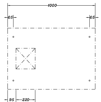
PLANTA PARA LOCALIZAÇÃO DE FIXAÇÃO, ENTRADA E SAÍDA DE CABOS, PARA COLUNAS SEM COMPARTIMENTO PARA CABOS
